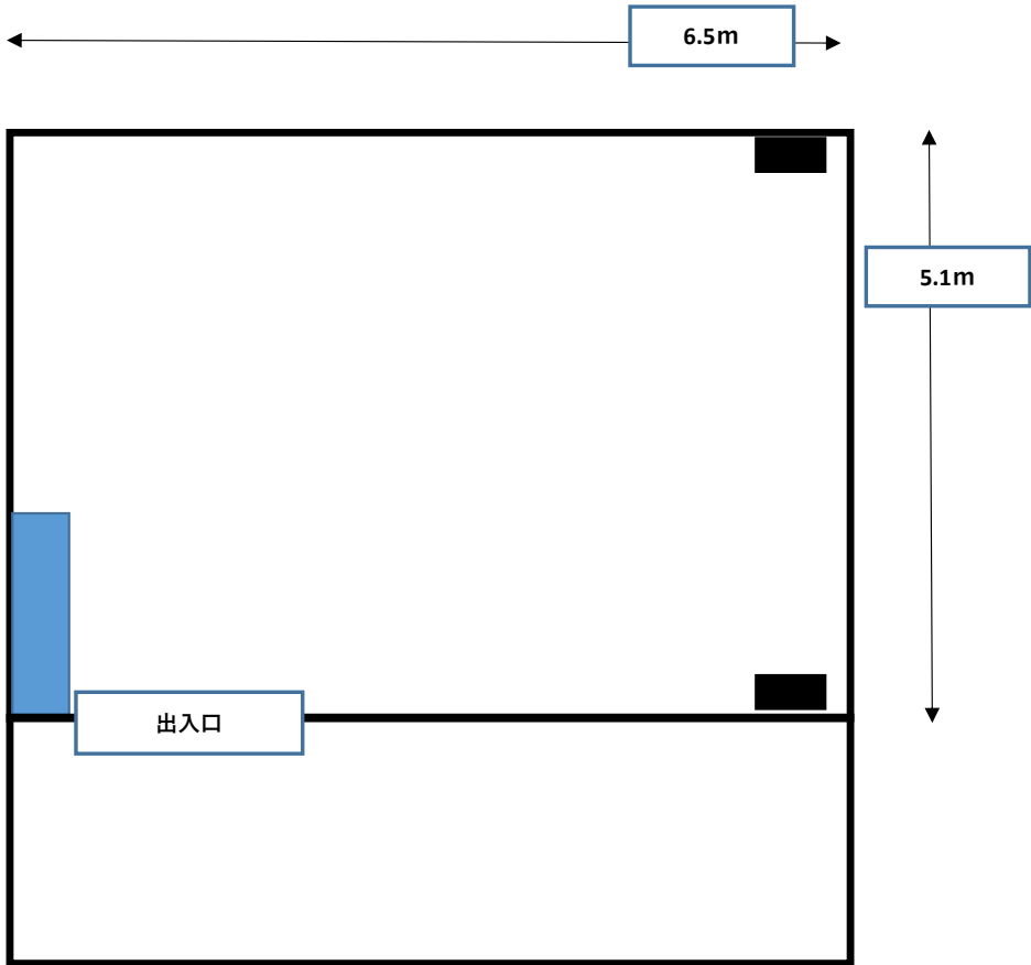
4-2 会議室 レイアウト
